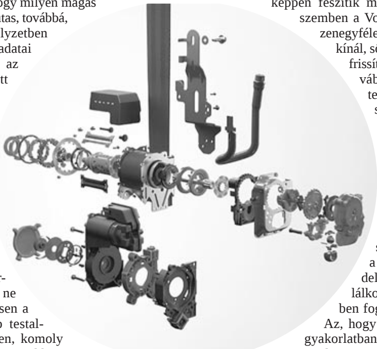
Volvo biztonsági öv rendszer Forrás: Volvo
